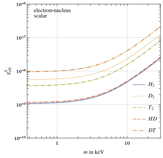
(d) Scalar electron–nucleus interaction with positive coupling g_{eN}^S > 0 .
